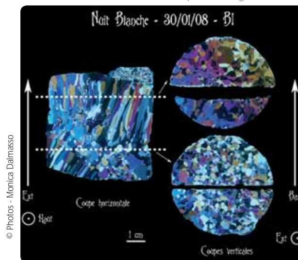
Observation d'une lame mince en lumière polarisée Observation of a thin section under polarized light
